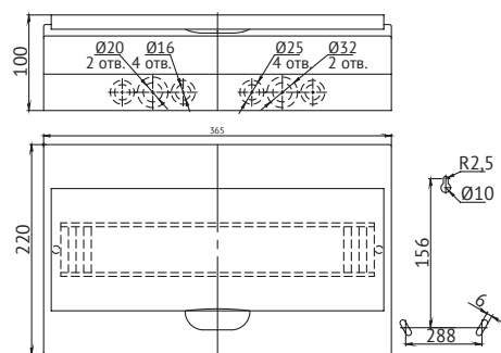
ЩРН-П-18-IP40
