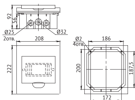
ЩРВ-П-8-IP40
