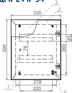
ЩРн-24 IP 54
