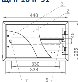
ЩРн-18 IP 31
