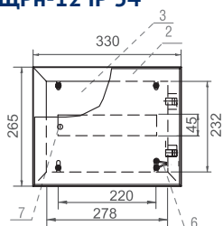
ЩРн-12 IP 54
