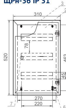
ЩРн-36 IP 31
