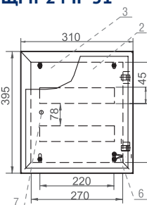
ЩРн-24 IP 31
