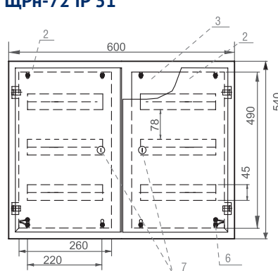
ЩРн-72 IP 31
