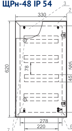
ЩРн-48 IP 54
