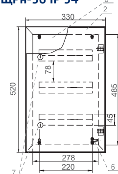
ЩРн-36 IP 54
