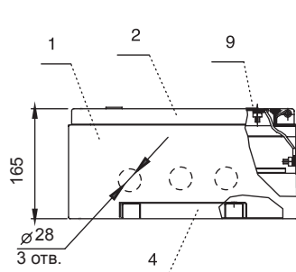
Панель ЩУРн-1/12-0, ЩУРн-3/12-0
