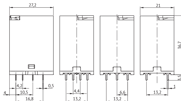
OptiRel G RP55-1X для монтажа на печатную плату с кнопкой тест
