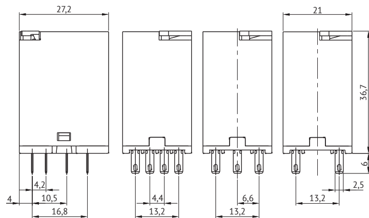
OptiRel G RP55-3X с кнопкой тест
