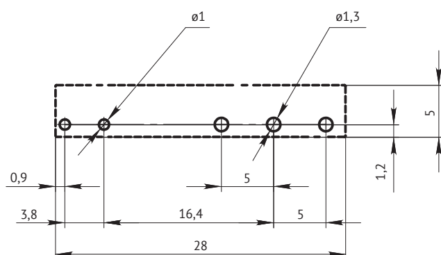
OptiRel G RP34 с СО контактами для монтажа на печатную плату
