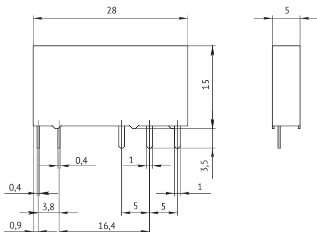
OptiRel G RP34 с СО контактами
