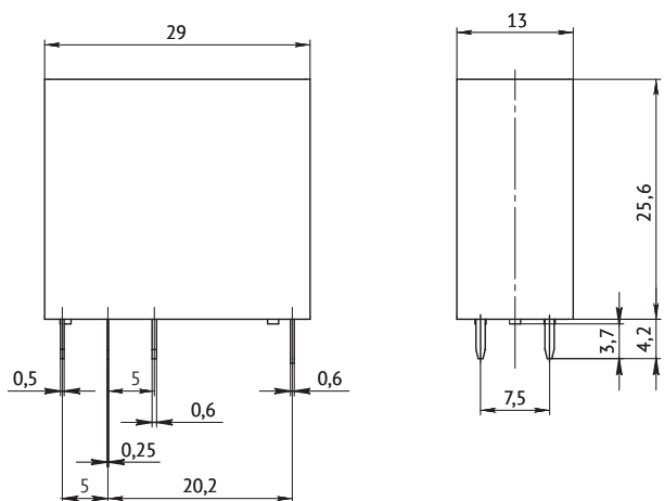
OptiRel G RP40-52 и OptiRel G RP40-61 с СО контактами
