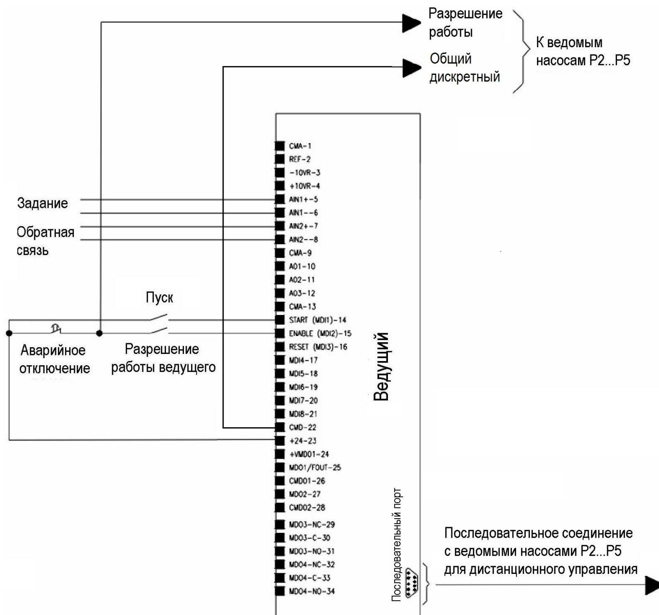
Рис. 11: Соединение ведущего привода с ведомыми по последовательной связи.
