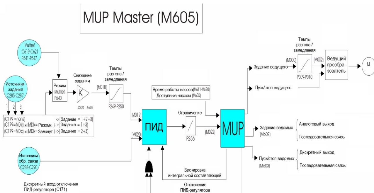
Рис. 2: Блок-схема OPTICOR P, работающего в режиме ведущего в насосной станции.
