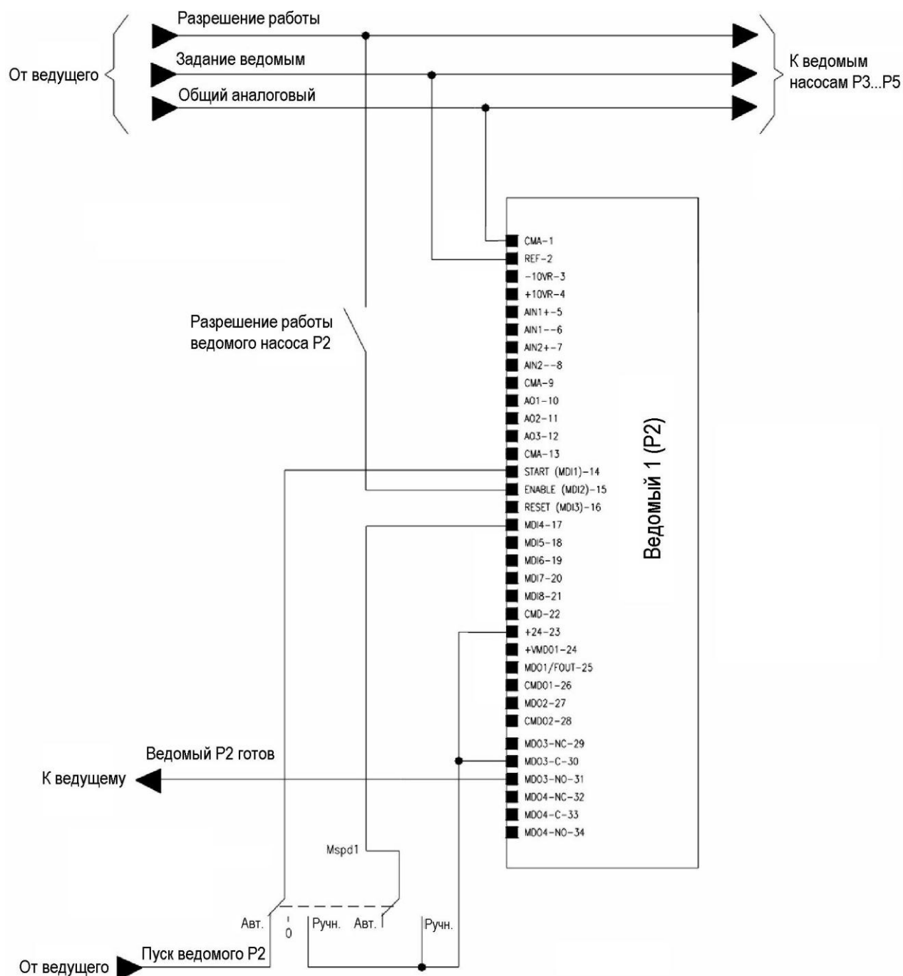
Рис. 10: Подключение сигналов к ведомому преобразователю при наличии переключателя "Ручной / Автоматический" и использовании задания скорости, выбираемого сигналом на входе MDI4, запрограммированном для выбора фиксированного задания.
