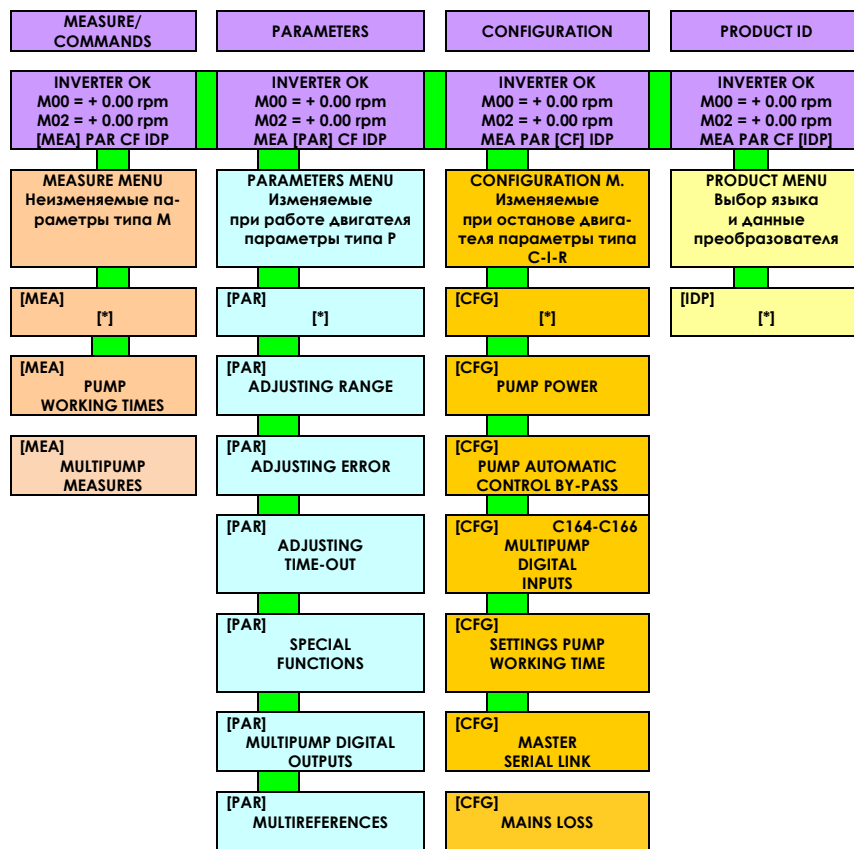
Рис. 14: Дерево меню.
