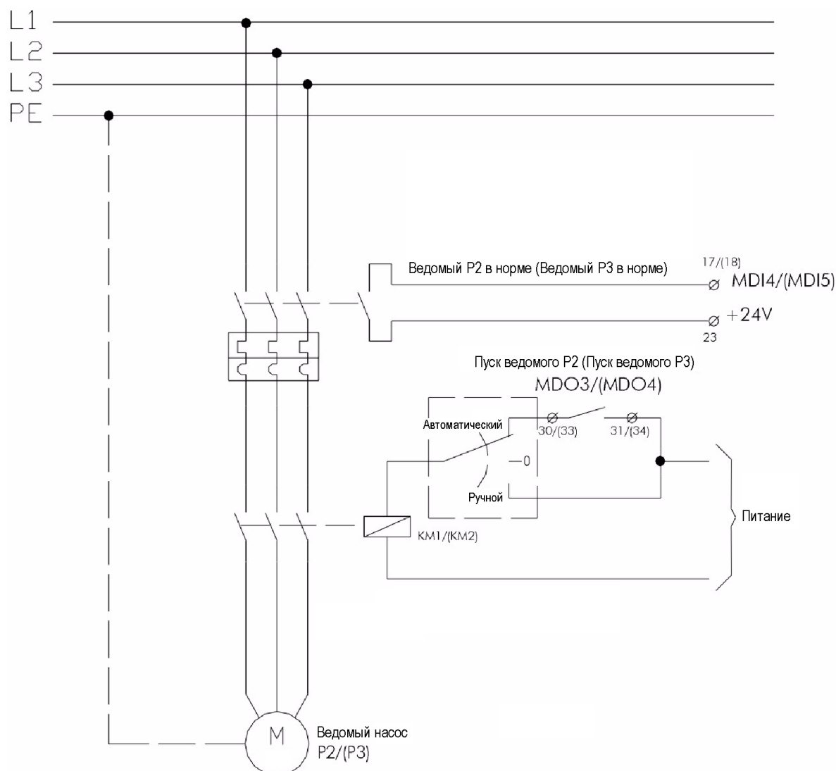
Рис. 4: Силовое подключение ведомых насосов P2 и P3
