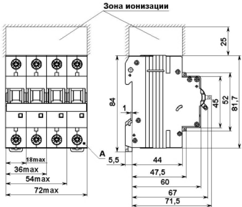
Рисунок Б.1 Габаритные, установочные и присоединительные размеры выключателей: Масса одного полюса не более 0,125 кг.
