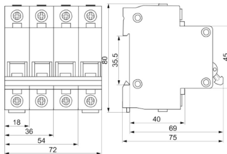
Рисунок В.1 Габаритные, установочные, присоединительные размеры выключателей.
