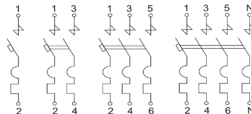
Рисунок Г.1 Принципиальные электрические схемы выключателей
