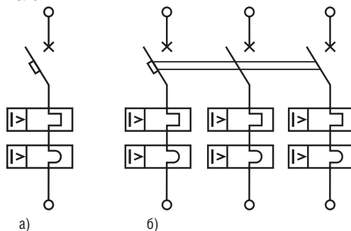
Рисунок Г.1. Принципиальные электрические схемы ограничителя:
