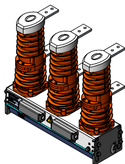
OptiMat BB-XX-XX/XXXX-Y2-1XX (базовое исполнение)
