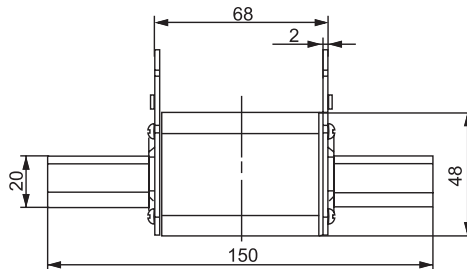
ППН-37 габарит 2 (40-250 А) масса 0,38 кг
