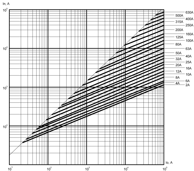
Рисунок Г.3 – Характеристики пропускаемого тока
