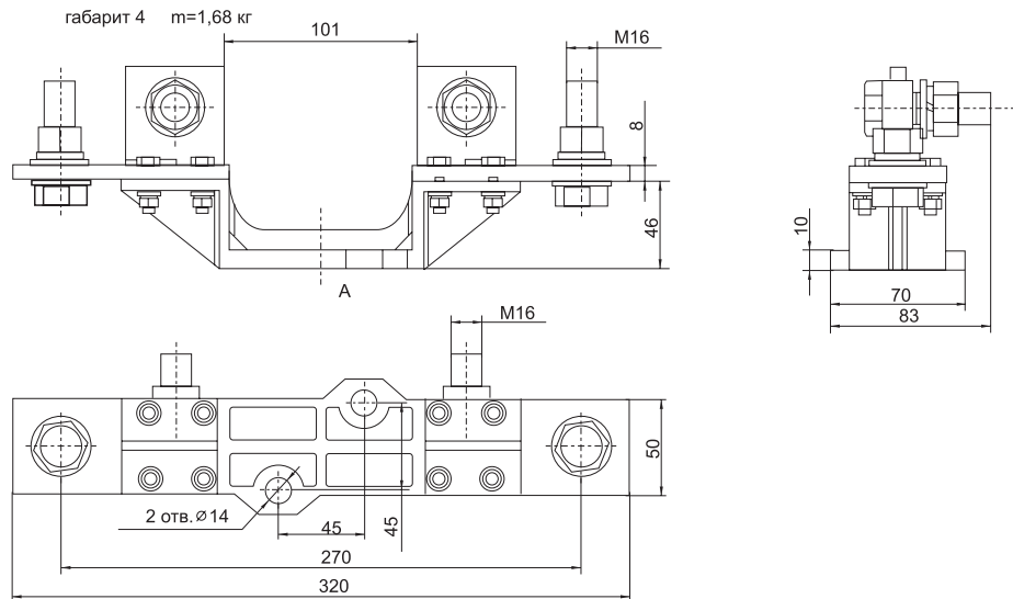
Рисунок В.7 – Основания (держатели) предохранителей ППН габариты 00, 0, 1, 2, 3, 4 исполнения 2
