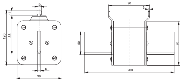
Рисунок В.3 – Плавкие вставки габаритов 4 и 4а
