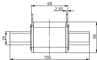
ППН-39 габарит 3 (100-400 А) масса 0,57 кг
