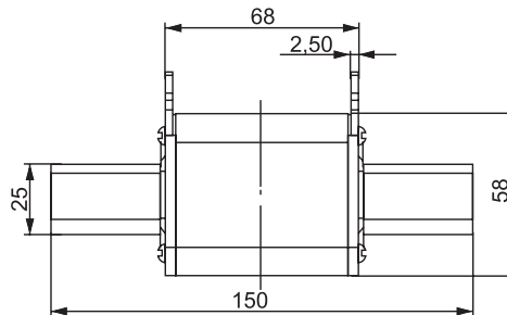
ППН-37 габарит 2 (315-400 А) масса 0,56 кг
