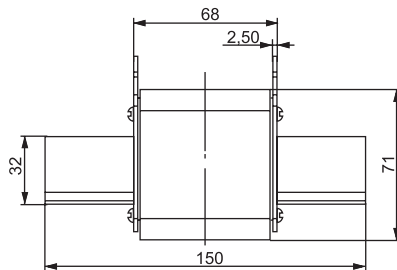
ППН-39 габарит 3 (500-630 А) масса 0,93 кг
