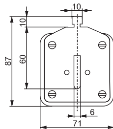
Рисунок В.2 – Плавкие вставки габаритов 2, 3
