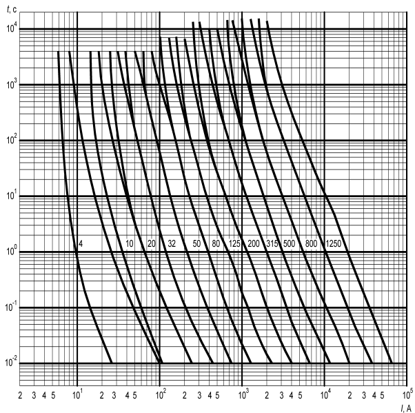
Рисунок Г.2 - Зона время-токовых характеристик
