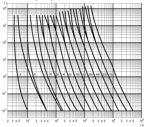
Рисунок Г.1 – Зона время-токовых характеристик
