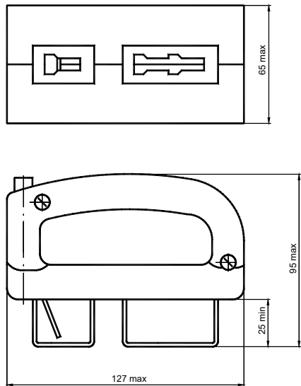
Рисунок В.8 – Рукоятка съема для смены плавких вставок Типоисполнение ППН/ПН2-Ф-УХЛ3-КЭАЗ
