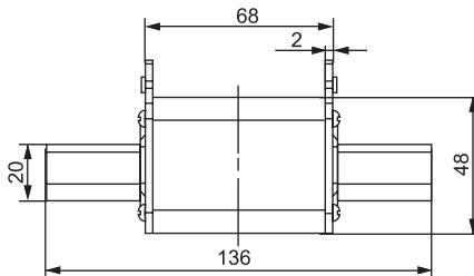
ПНН-35 габарит 1 (200-250 А) масса 0,36 кг
