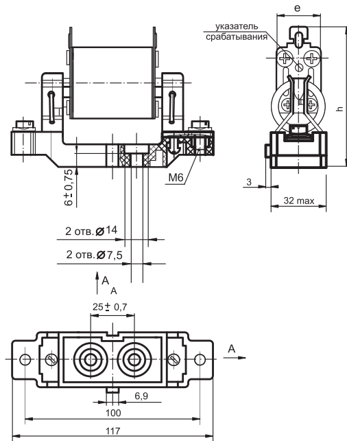
Рисунок В.4 – Основания (держатели) предохранителей ППН Габарит 00, исполнение 1В
