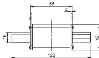
ППН-33 габарит 0 масса 0,2 кг
