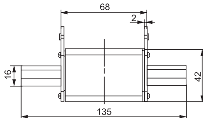
ПНН-35 габарит 1 (6-160 А) масса 0,23 кг
