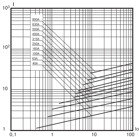
I_o - ток отключения, кА I - ток, пропускаемый предохранителем, кА Рисунок В.15. Предохранители типа ПП57-3167, ПП57-3467, ПП57-3767, ПП57-3967, ПП57-3768, ПП57-3968, ПП57-4068, ПП57-3968Б
