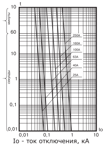
Рисунок В.1. Предохранители типа ПП57-3427
