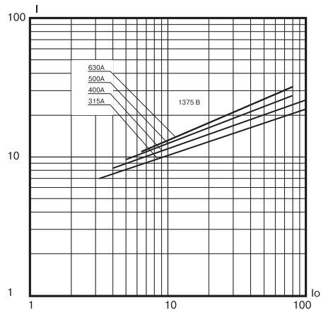
I_o - ток отключения, кА I - ток, пропускаемый предохранителем, кА Рисунок В.15. Предохранители типа ПП57-3797, ПП57-3997, ПП57-3998К, ПП57-3998
