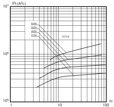
I_0 - ток отключения, кА Рисунок В.12. Предохранители типа ПП57-3797, ПП57-3997, ПП57-3998К, ПП57-3998
