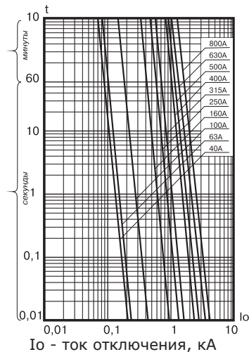
Рисунок В.2. Предохранители типа ПП57-3137, ПП57-3437, ПП57-3737, ПП57-3937, ПП57-3738, ПП57-3938, ПП57-4038
