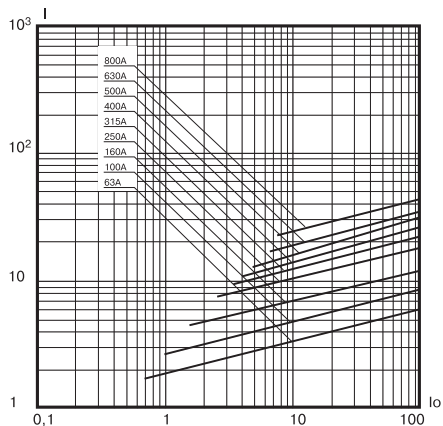
I_0 - ток отключения, кА I - ток, пропускаемый предохранителем, кА Рисунок В.14. Предохранители типа ПП57-3137, ПП57-3437, ПП57-3737, ПП57-3937, ПП57-3738, ПП57-3938, ПП57-4038
