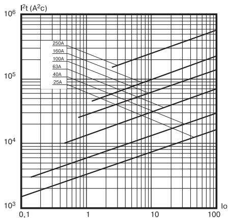
Рисунок В.9. Предохранители типа ПП57-3427
