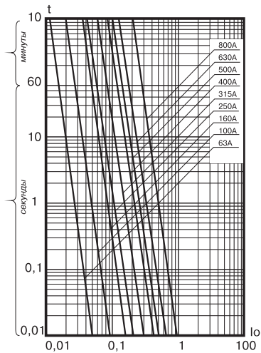
Рисунок В.3. Предохранители типа ПП57-3167, ПП57-3467, ПП57-3767, ПП57-3967, ПП57-3768, ПП57-3968, ПП57-4068, ПП57-3968Б
