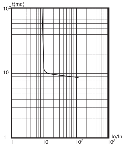
I_o/I_{ном} - отношение тока отключения (действующее значение) к номинальному Рисунок В.8. Предохранители типа ПП57-3797, ПП57-3997, ПП57-3998К, ПП57-3998
