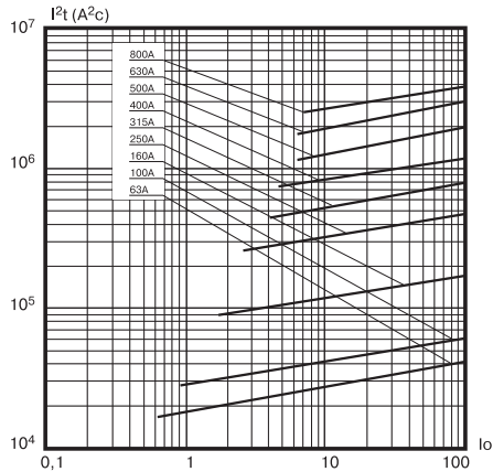
I_0 - ток отключения, кА Рисунок В.11. Предохранители типа ПП57-3167, ПП57-3467, ПП57-3767, ПП57-3967, ПП57-3768, ПП57-3968, ПП57-4068, ПП57-3968Б
