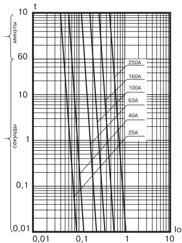
Рисунок В.5. Предохранители типа ПП57-3427
