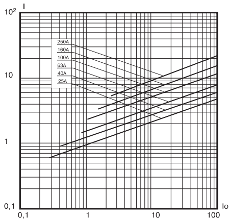
I_0 - ток отключения, кА I - ток, пропускаемый предохранителем, кА Рисунок В.13. Предохранители типа ПП57-3427
