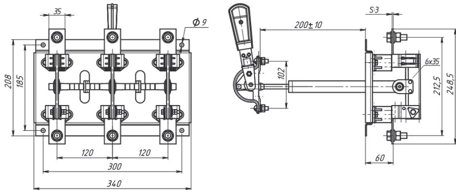
Рисунок Б.8 - Разъединитель серии Р с центральным приводом РС-6 на номинальный ток 630 А
