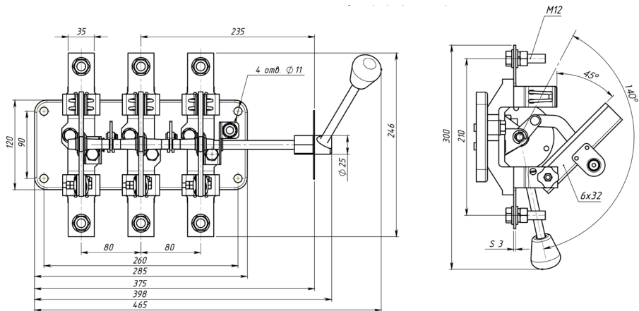
Рисунок Б.5 - Разъединитель серии Р с боковой рукояткой РБ-6 на номинальный ток 630 А
