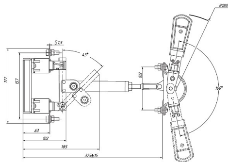
Рисунок Б.6 - Разъединитель серии Р с центральным приводом РЦ-1 на номинальный ток 100 А
