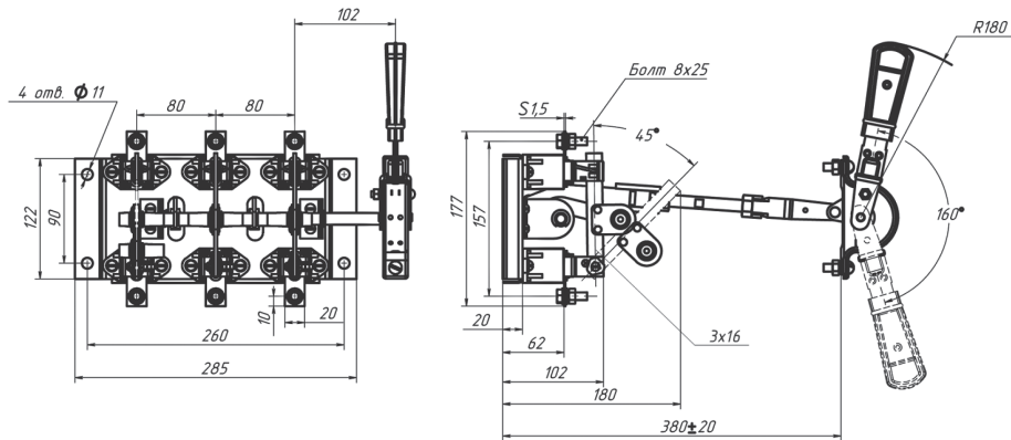
Рисунок Б.1 - Разъединитель серии Р с передней смещенной рукояткой РС-1 на номинальный ток 100 А
