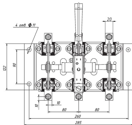
Рисунок Б.6 - Разъединитель серии Р с центральным приводом РЦ-1 на номинальный ток 100 А
