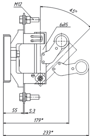
Рисунок Б.9 - Разъединитель Р43 с пополюсным оперированием штангой ШО-1 на номинальный ток 250 А и 400 А
