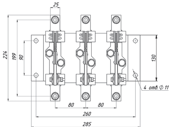
Рисунок Б.10 - Разъединитель Р63 с полюсным оперированием штангой ШО-1 на номинальный ток 630 А
