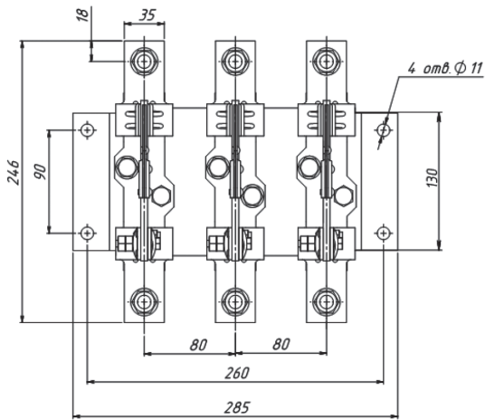
Рисунок Б.9 - Разъединитель Р43 с пополюсным оперированием штангой ШО-1 на номинальный ток 250 А и 400 А
