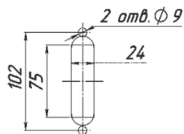
Рисунок Б.2 - Разъединитель серии Р с передней смещенной рукояткой PC-2, PC-4, PC-6 на номинальный ток 250 А, 400 А и 630 А
