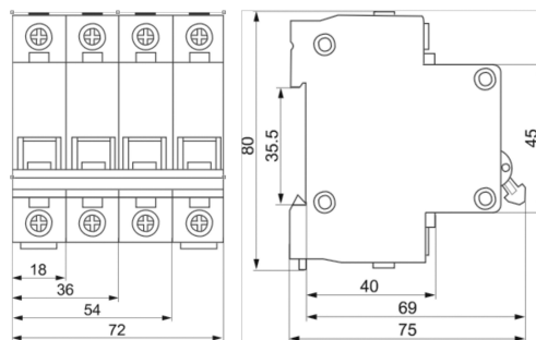
Рисунок Б.1 Габаритные, установочные, присоединительные размеры выключателей.
